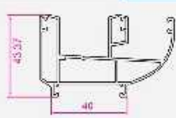
فریم کشویی KP617
