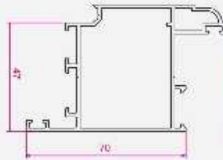
لنگه درب لولایی KP585
