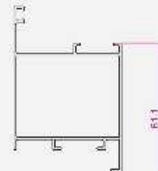
لنگه سنگین درب KP527
