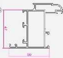
لنگه پنجره لولایی KP586
