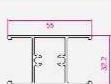
سپری کشویی KP619
