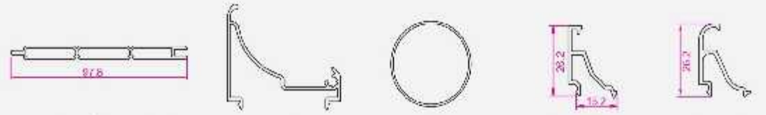
فاساد دو خط تک جداره KP511 ناخن KP565 لوله KP566 زهوار دو جداره KP560 زهوار دو جداره KP561
